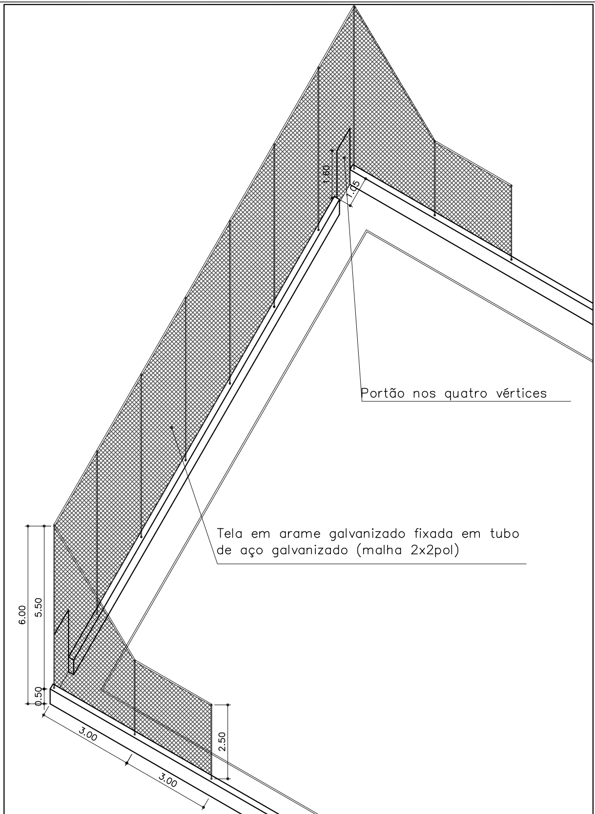
PERSPECTIVA TELA (QUADRA) ESCALA.....1/125
